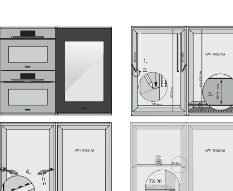
Schemi per KWT 6422 iG
