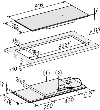
KM 7684 FL installazione in appoggio
